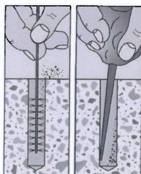
Bohrloch reinigen
