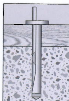
Dübel einstecken
